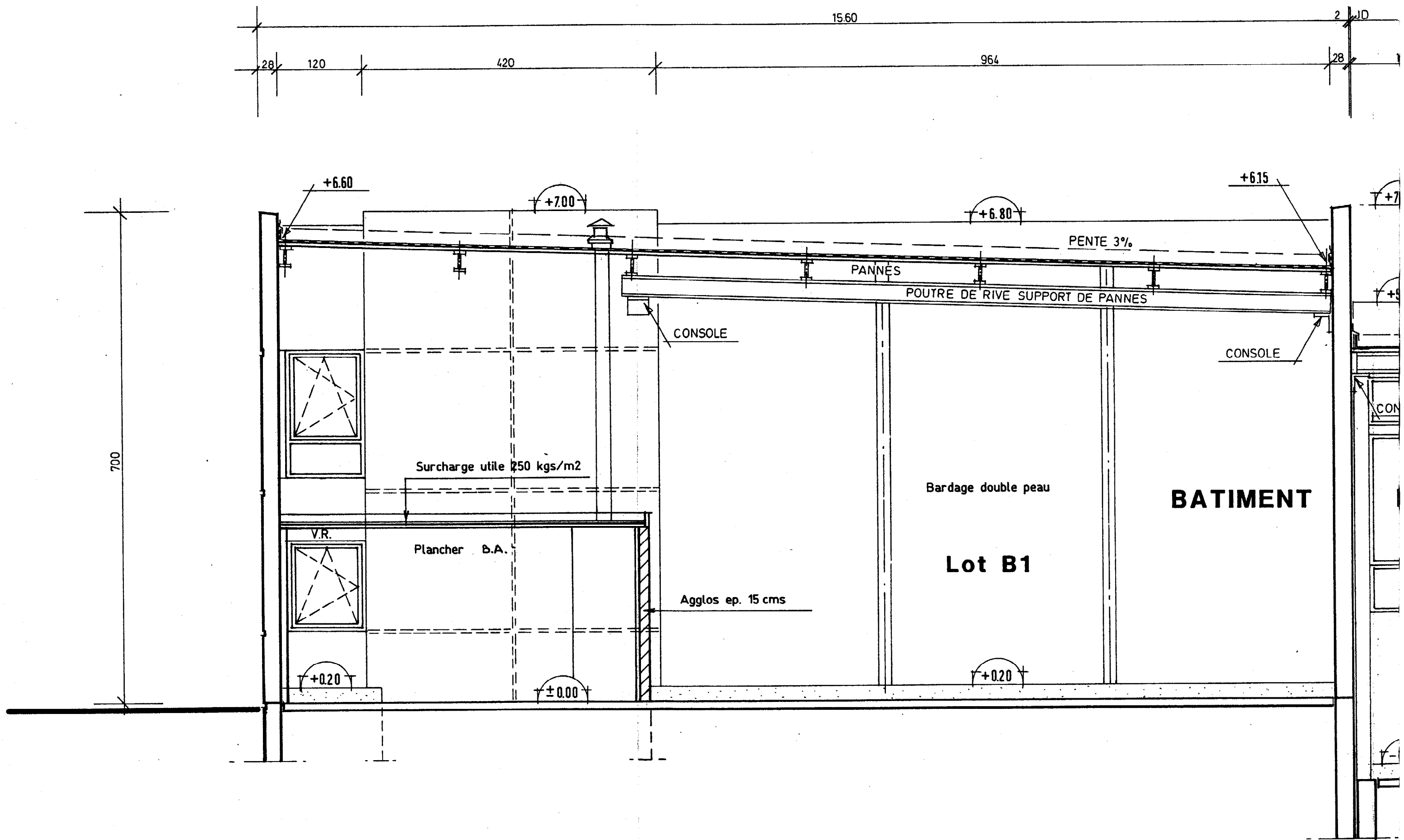
COUPE B-
