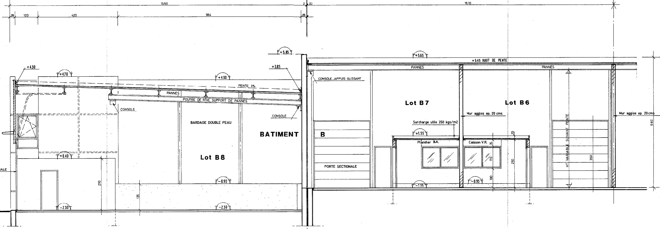
COUPE C-C
