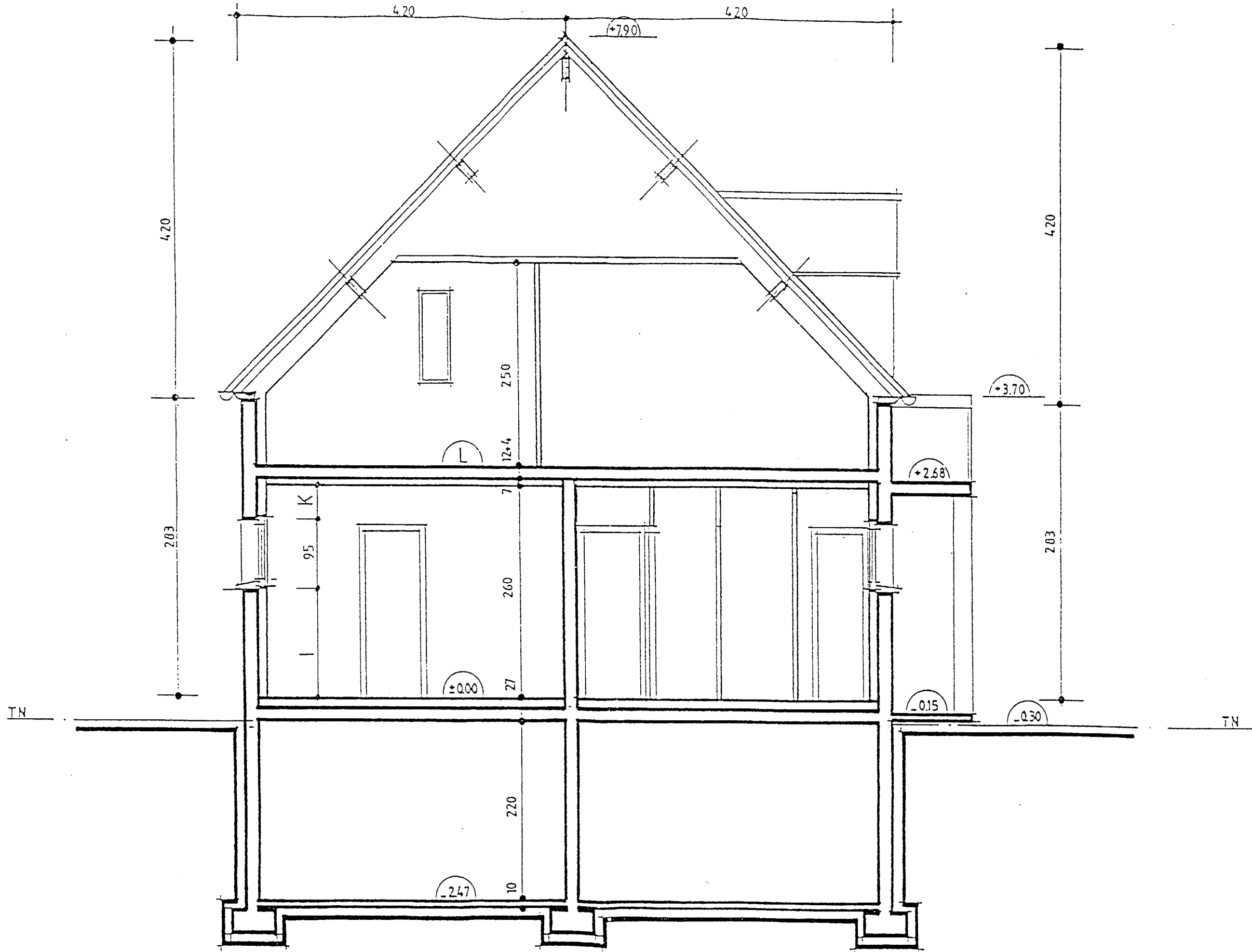
COUPE AA
