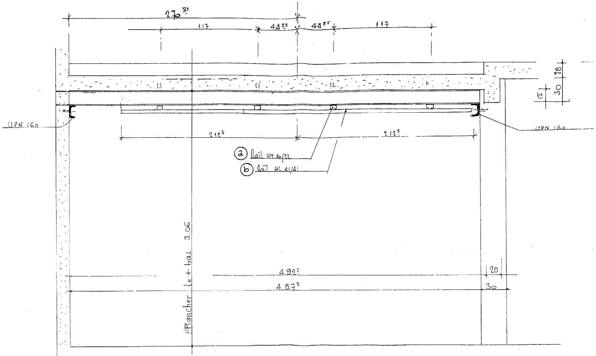
COUPE 1.1
