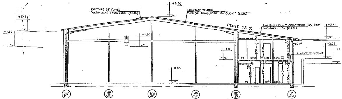
COUPE A-A
