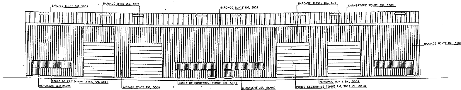
FACADE NORD
