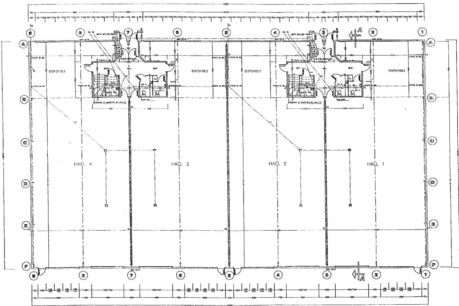
PLAN A3
