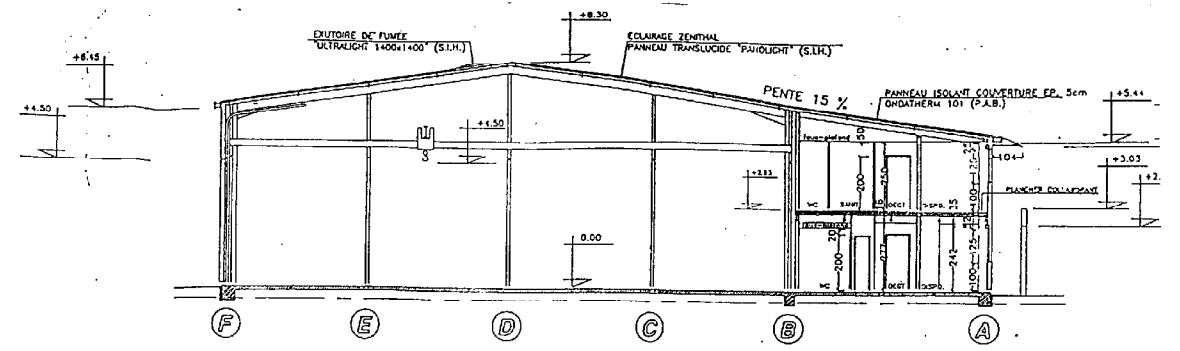
COUPE A-A
