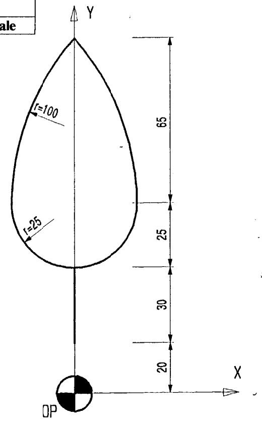
Détail échelle 2:1
