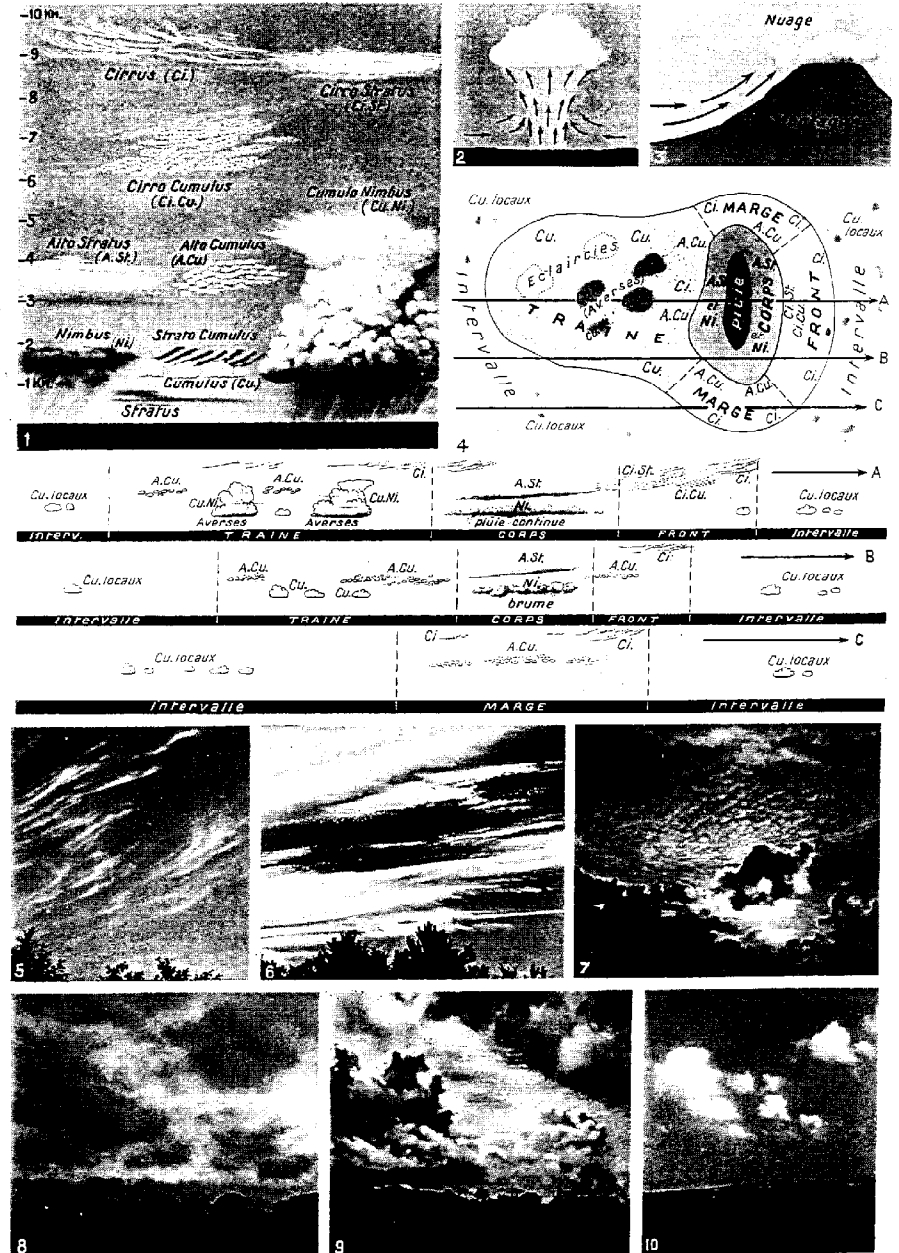
NUAGES II. — 1. Altitudes moyennes des divers nuages ; 2 et 3. Formation de nuages par mouvement ascensionnel de l'air déterminant la condensation de la vapeur d'eau ; 4. Schématisation d'un système nuageux ; plan de la distribution des diverses formations stratiformes et, au-dessous, succession de leur passage suivant les trois coupes A, B, C. Ciel révélant la proximité d'un système nuageux ; 5. Ciel de front ; 7. Ciel de marge ; 8. Ciel de train ; 9. Ciel de corps ; 10. Ciel d'intervalle.
