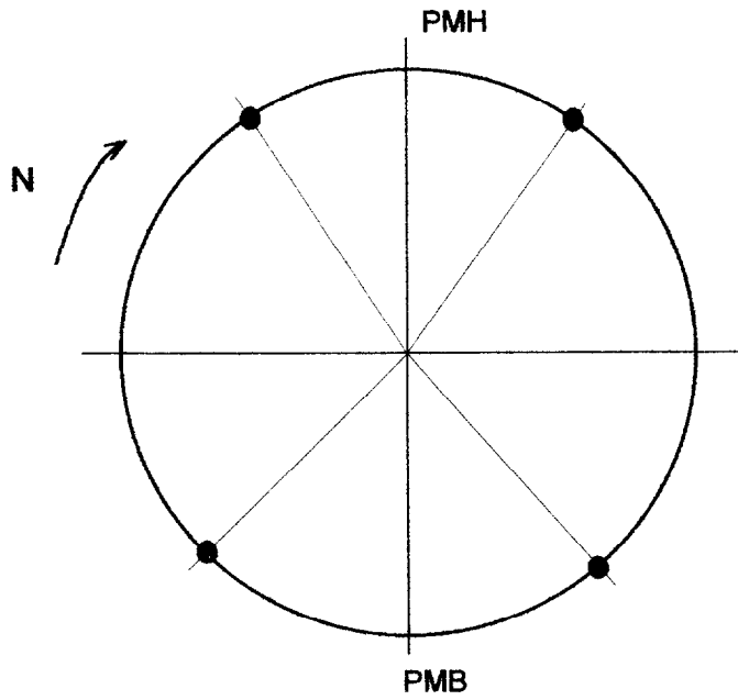
12 : Diagramme circulaire de distribution
