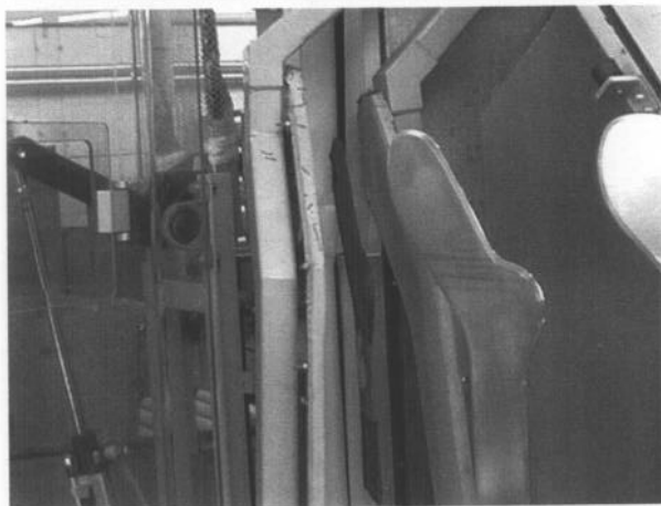
"MULTIJOB": formage automatique de la chaussette entre 2 presses
