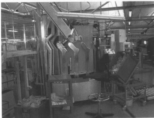
"MULTIJOB": zone d'enfilage des chaussettes sur les gabarits et contrôle après formage
