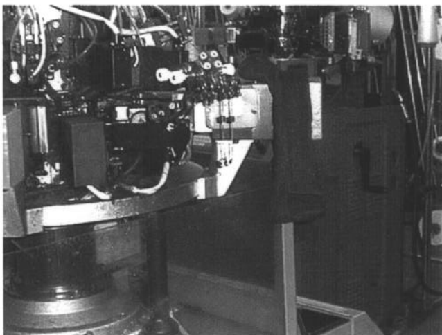
Chaussette "tombée" du métier, pointe ouverte
