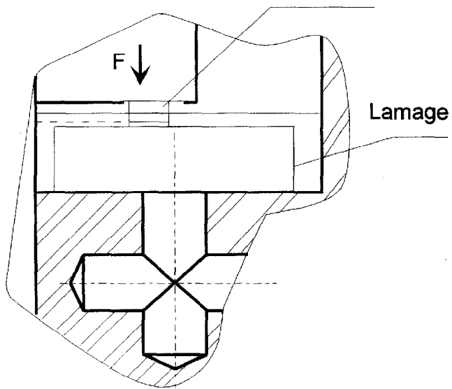
Détail Ech 8:1 (piston en position basse) Rainure circulaire
