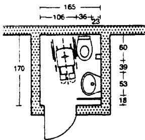
WC pour handicapé moteur.
