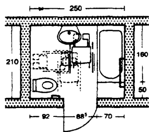
Dimensions d'une salle d'eau.
