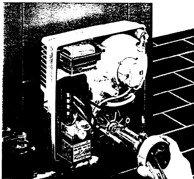
Accessibilité de la chambre de mélange sur les types WG1 et WG2
