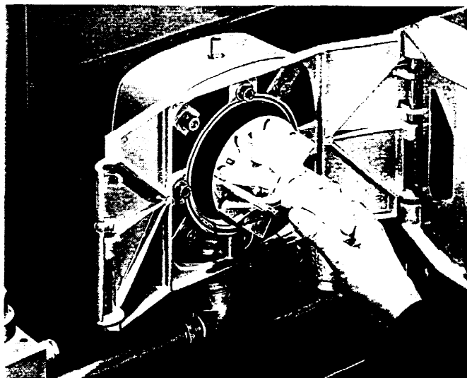
Accessibilité de la chambre de mélange sur les types WG1 et WG2
