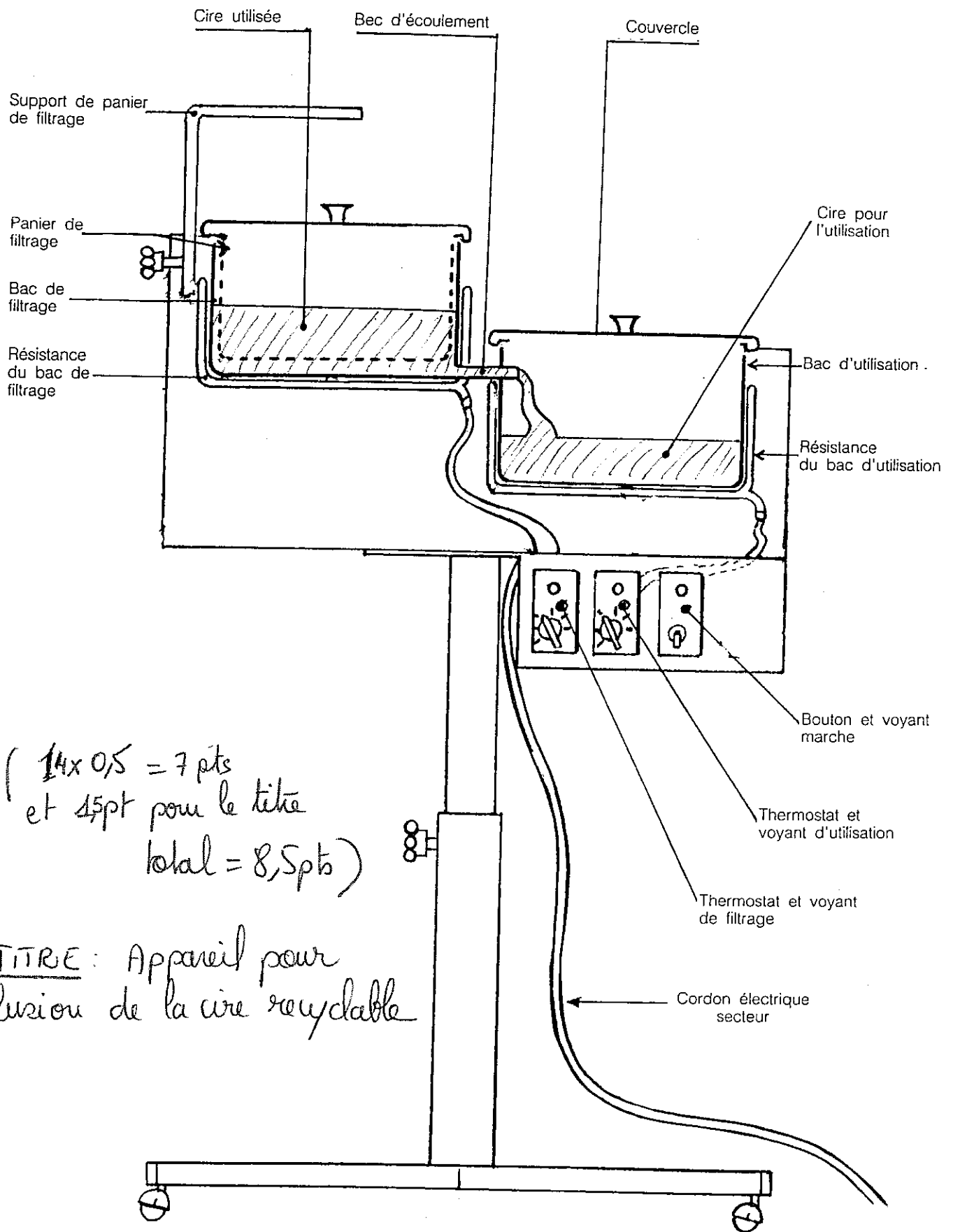
Schéma exécuté d'après l'appareil « FLUVITA »
