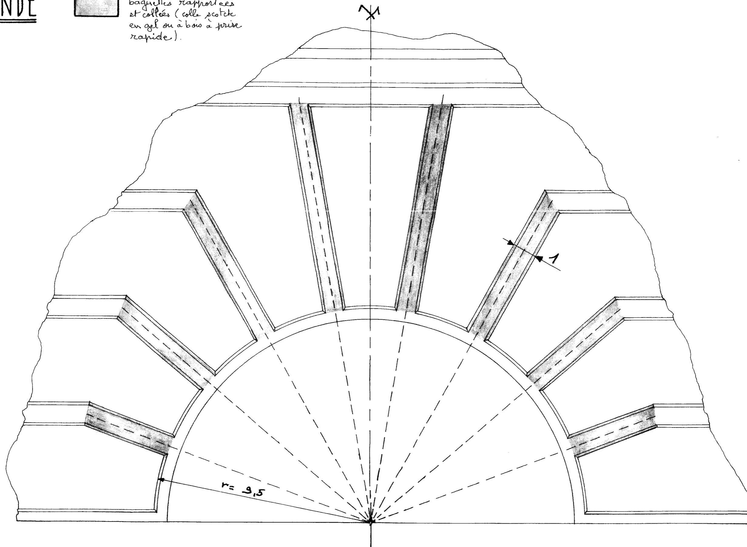
DETAIL B ÉCH: 1/1
