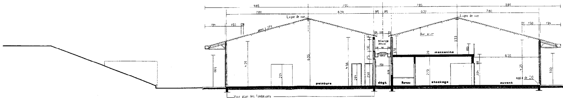
COUPE AA
