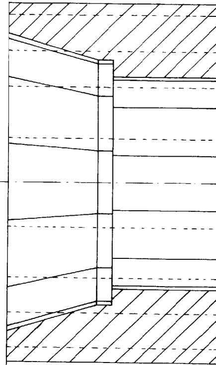
COUPE DD
