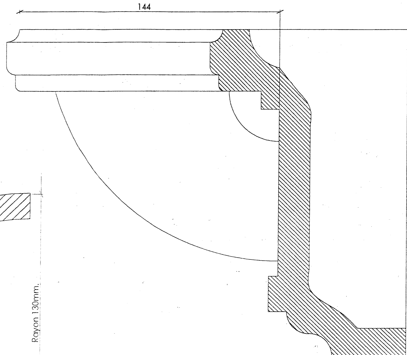
COUPE A-A (1:1)
