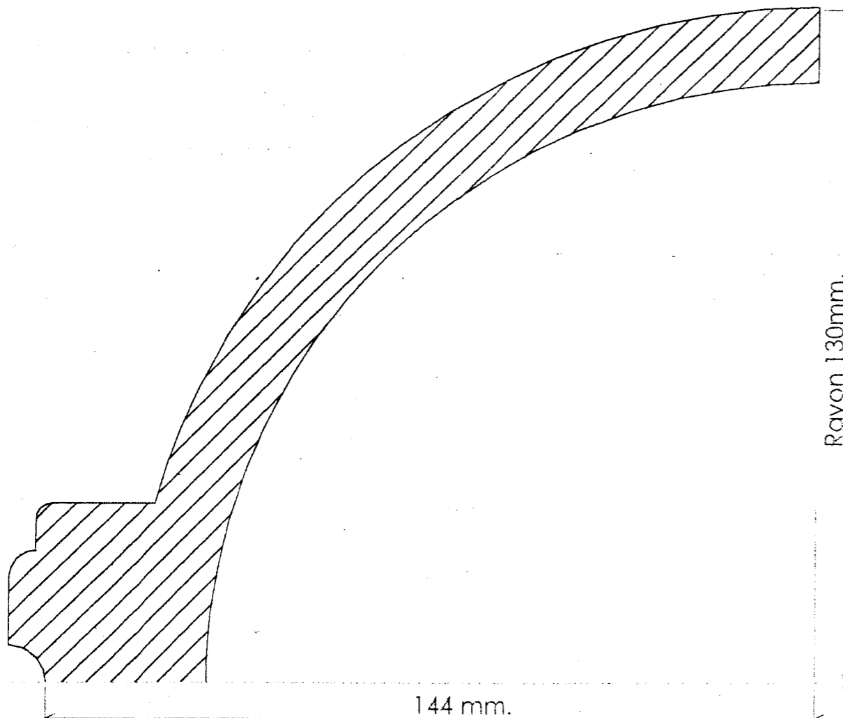
PROFIL APPLIQUE (1:1)
