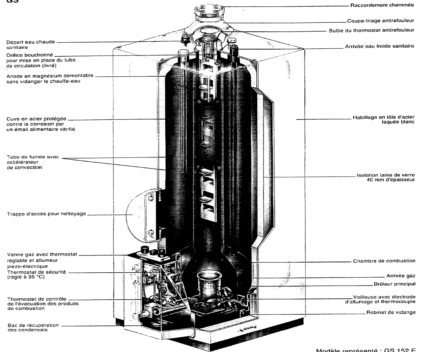
Modèle représenté : GS 152 E
