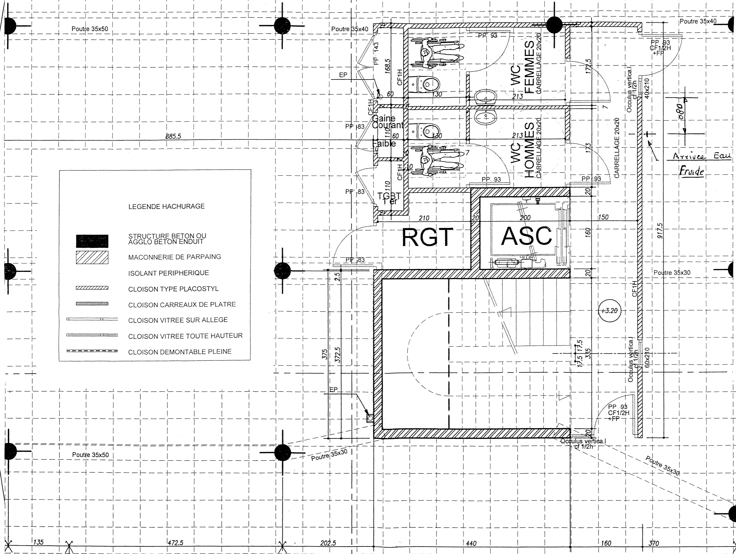
PLAN Modification du 1° étage; Traçage au crayon bleu.
