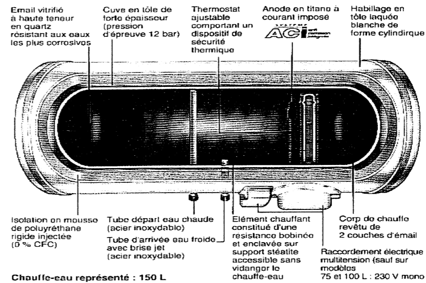
Chauffe-eau représenté : 150 L
