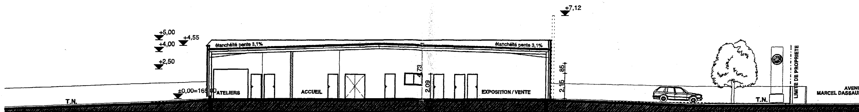
COUPE TRANSVERSALE A-A COUPE PAYSAGÈRE
