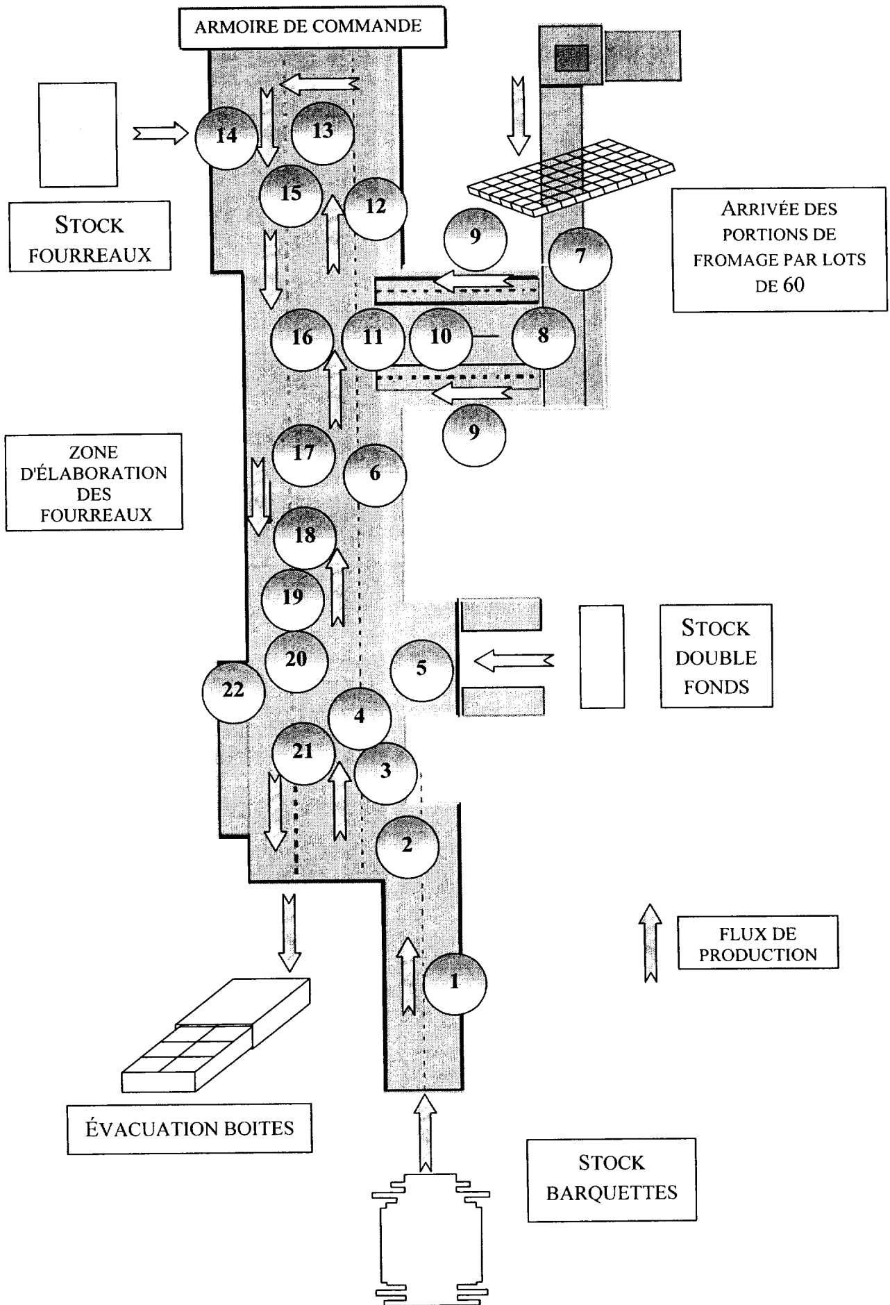
SCHÉMA D'IMPLANTATION DU SYSTÈME CONDITIONNEMENT DE FROMAGES (VUE DE DESSUS)
