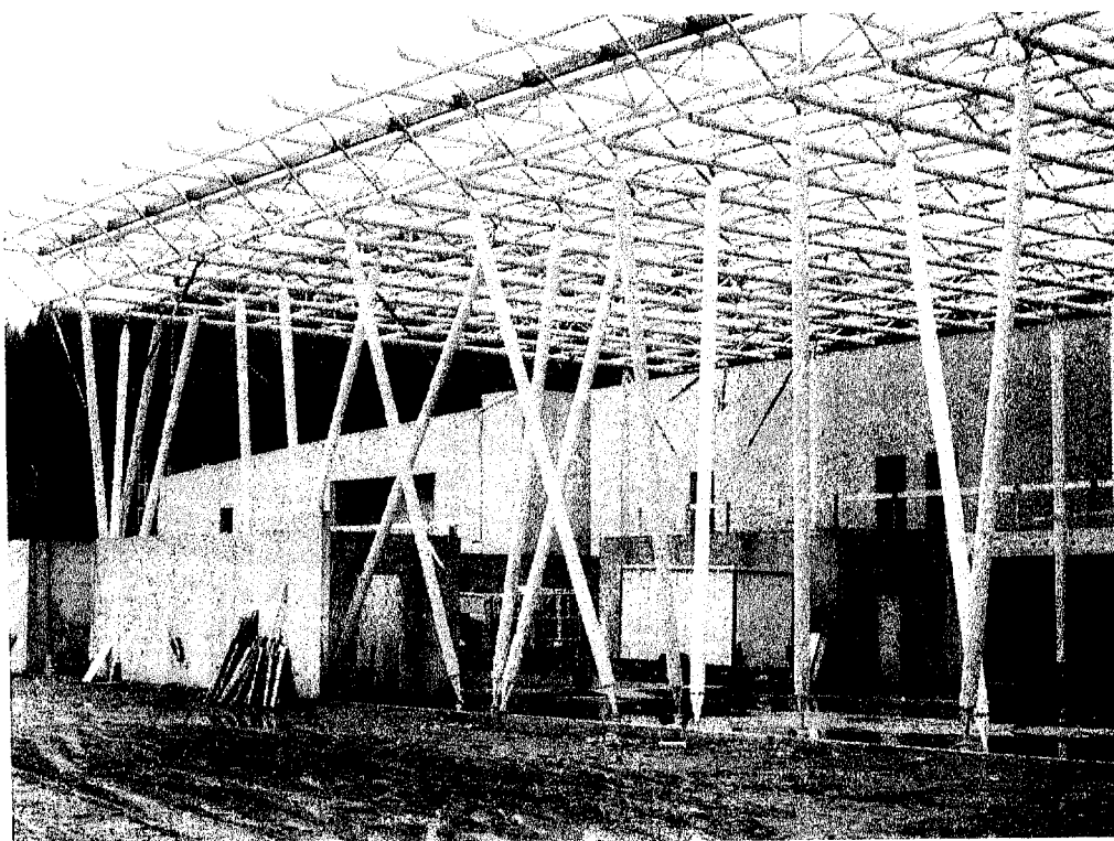
FACADE NORD - EST : NAPPE 3D ET POTEAUX MIKADOS
