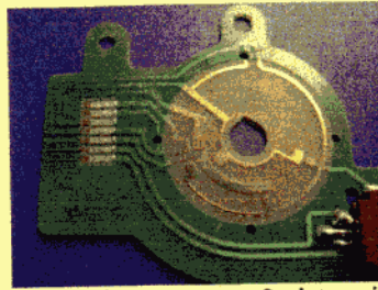
Circuit imprimé comportant 3 pistes circulaires cuivrées.
