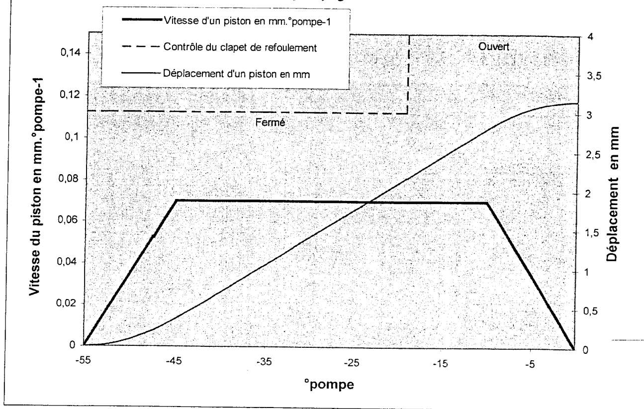
Diagramme de pompage avec actuateur BP
