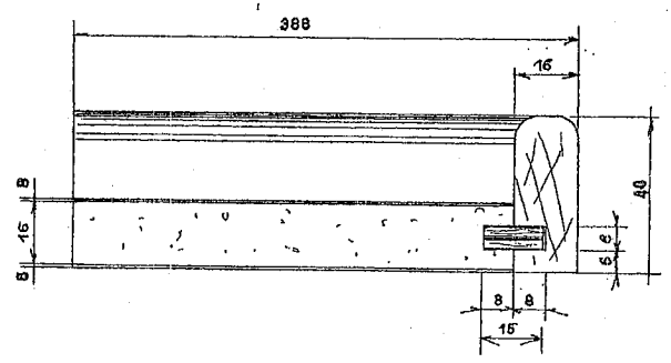
DETAIL ETAGERE
