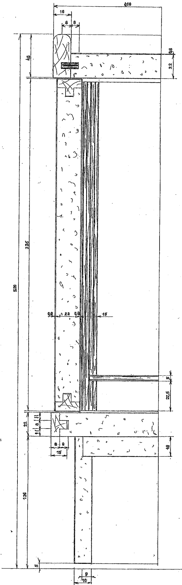
COUPE AA
