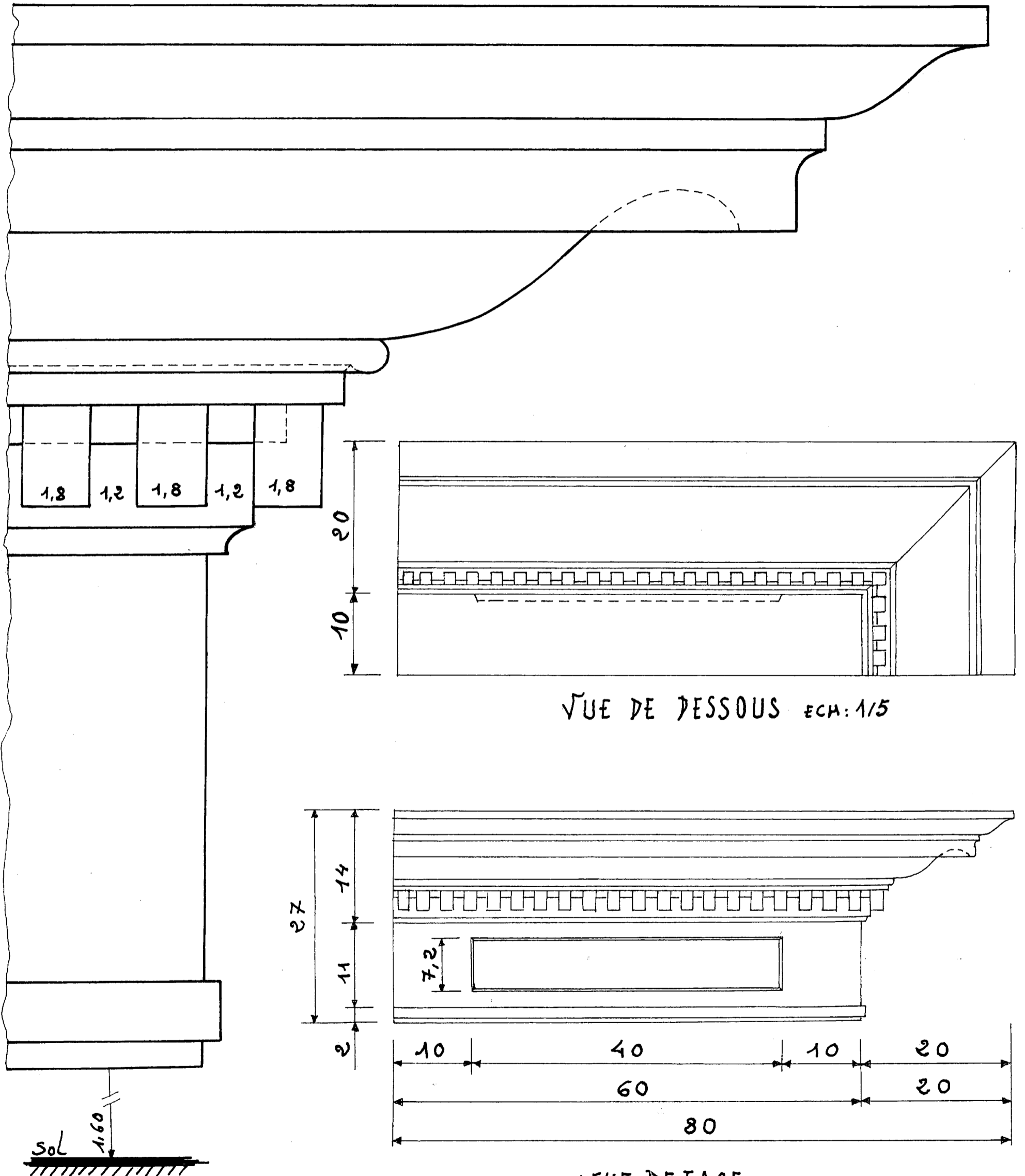
VUE DE FACE ECH: 1/5
