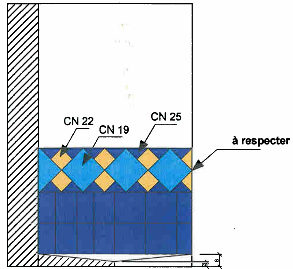
COUPE BB
