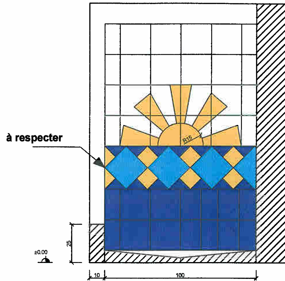
COUPE AA
