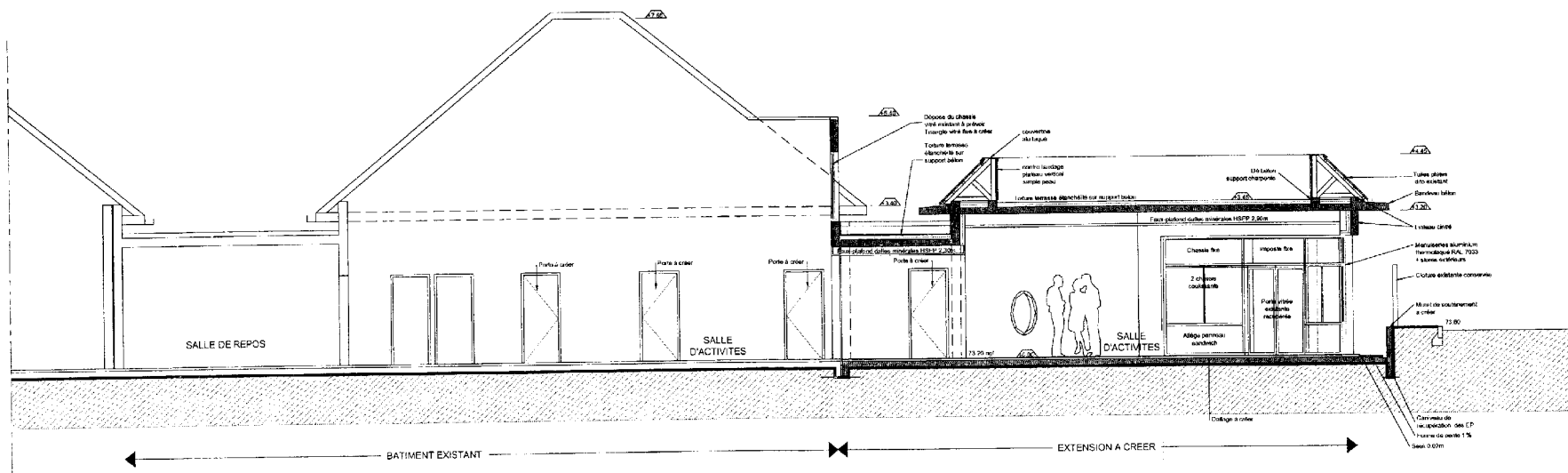
COUPE A-A
