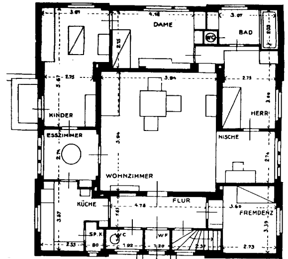
GRUNDRISS
