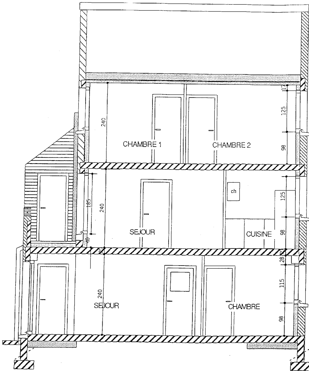
COUPE 5
