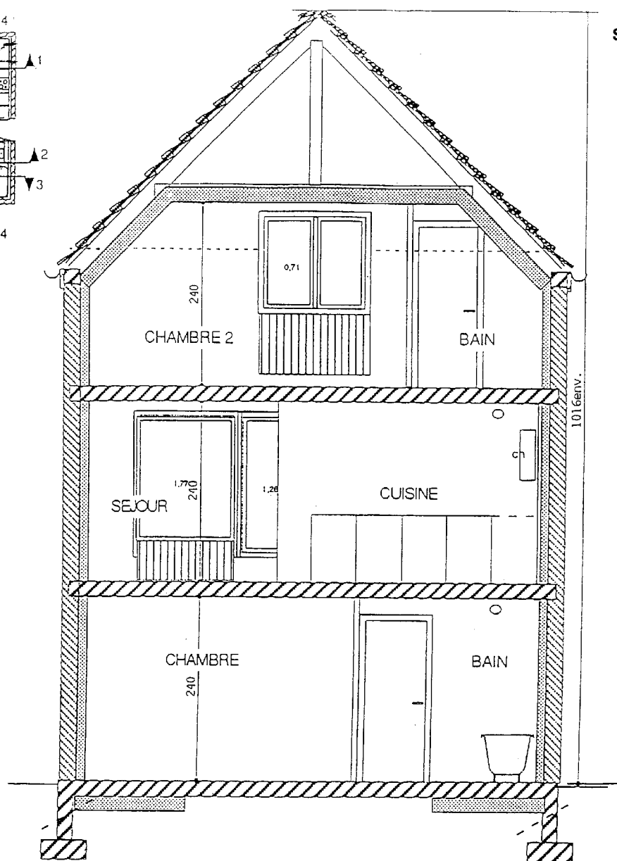
COUPE R.D.C
