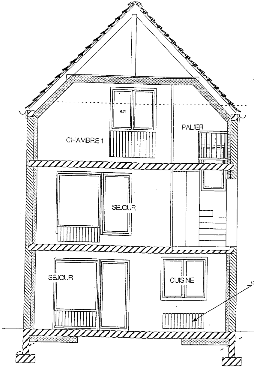
COUPE 1
