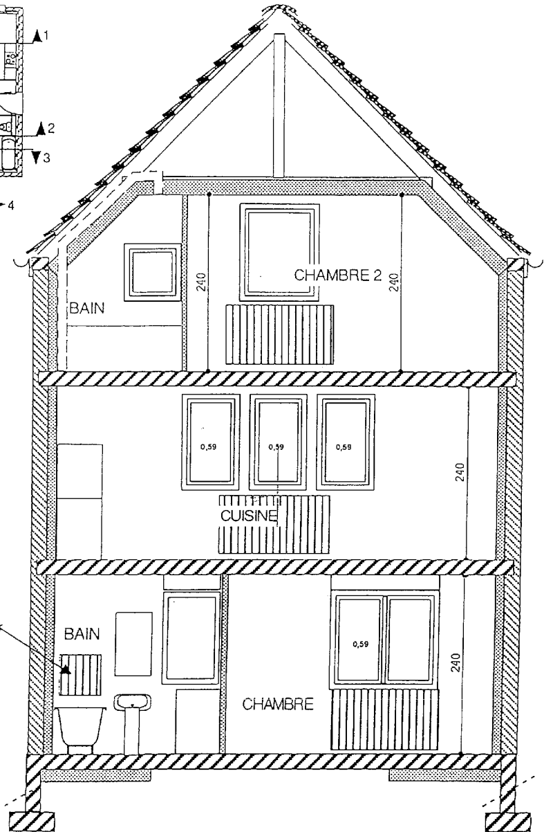
COUPE 3
