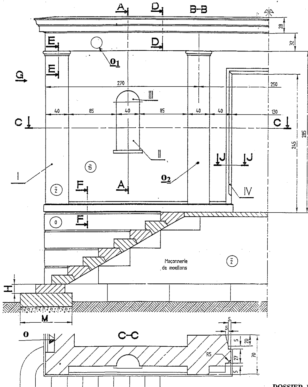
Echelle 1 : 25
