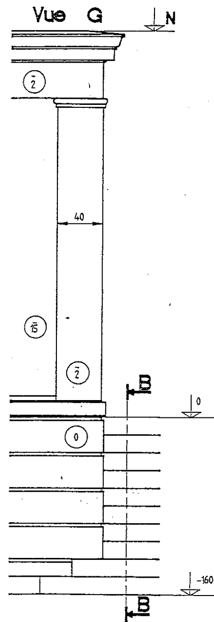
Echelle 1 : 25
