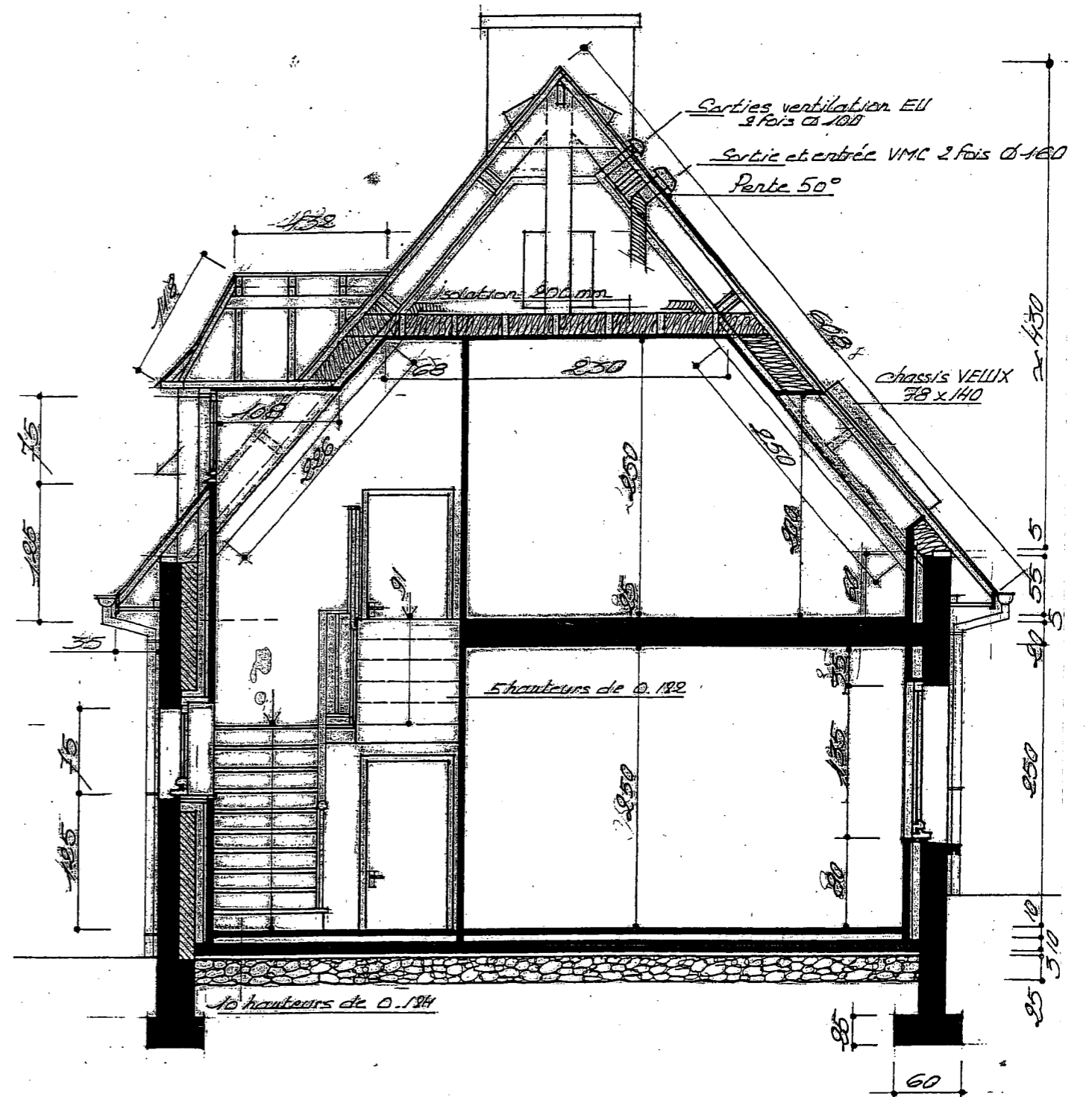
COUPE BB
