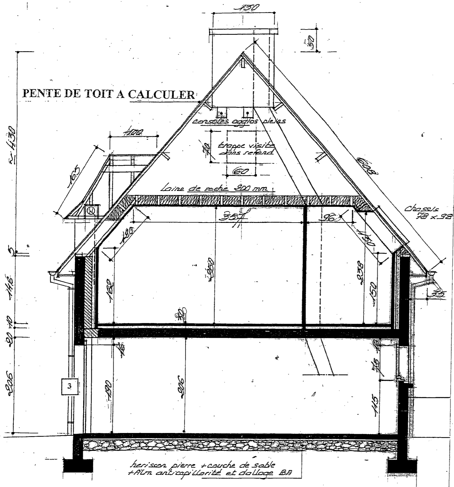
COUPE AA
