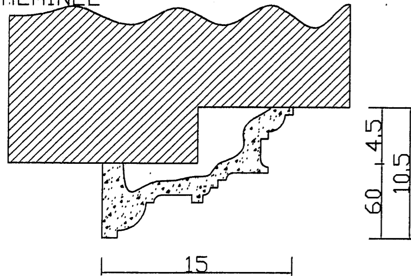
DETAIL DE LA MOULURE A DE LA CHEMINEE
