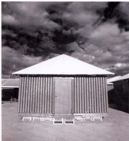
Document 4 : Shigeru BAN, Habitat pour réfugiés , Kobé, Japon, 1995. Tubes de carton, caisses de bières lestées de sable, contreplaqué, toile téflon.
