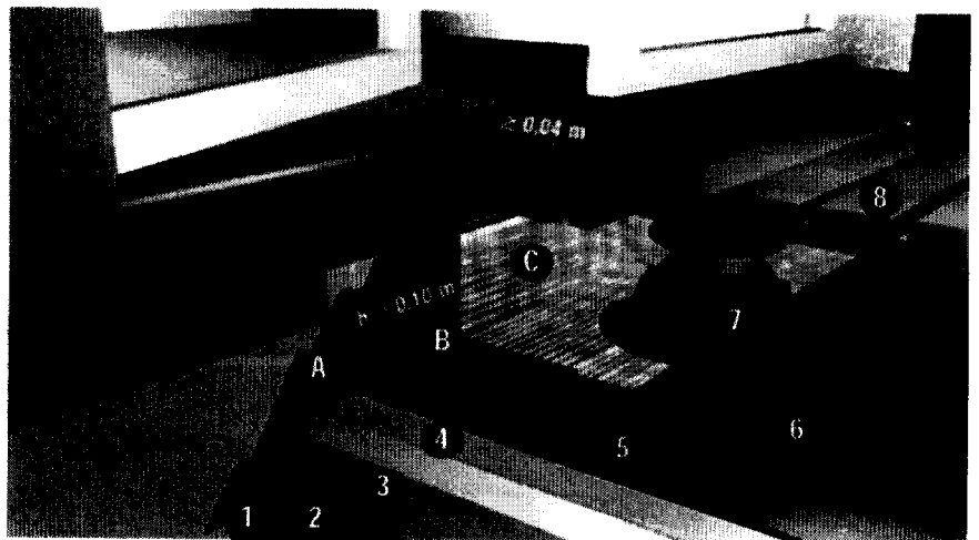
1. Primaire 2. Pare-vapeur 3. Isolant 4. SOPRAVOILE 100 5. SOPRALENE FLAM 100 6. ELASTOPHENE FLAM 25 7. Plot à verin SOPREMA 8. DALDECOR
