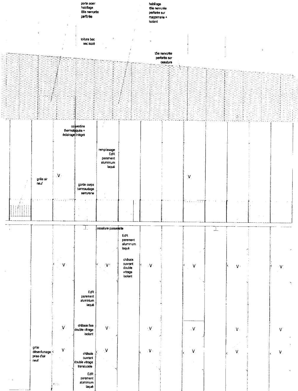
Détail façade ouest
