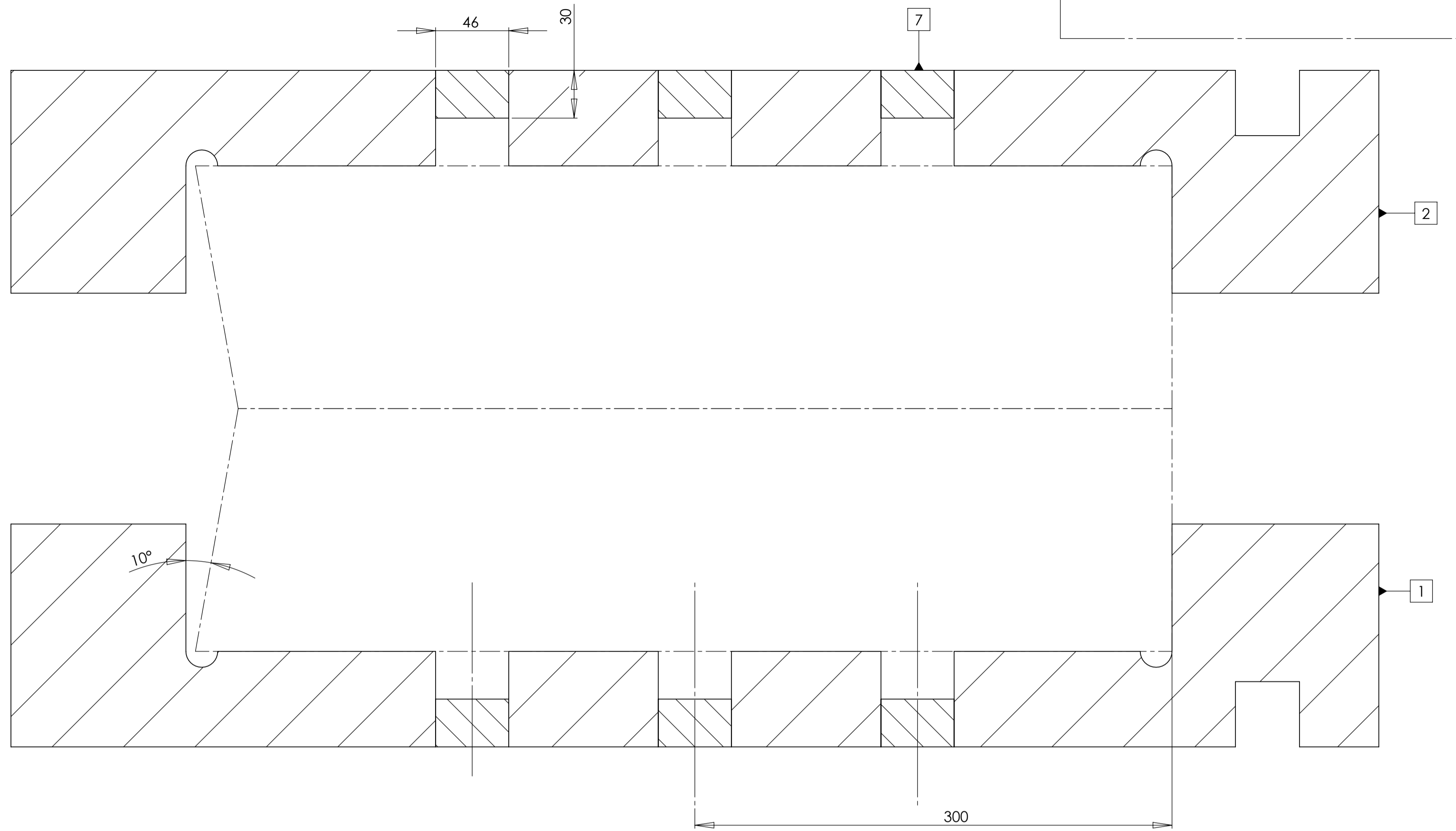
SECTION A-A ECHELLE 1 : 2
