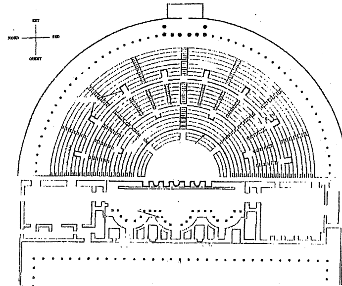
PLAN DU THEATRE ROMAIN D'ARLES
