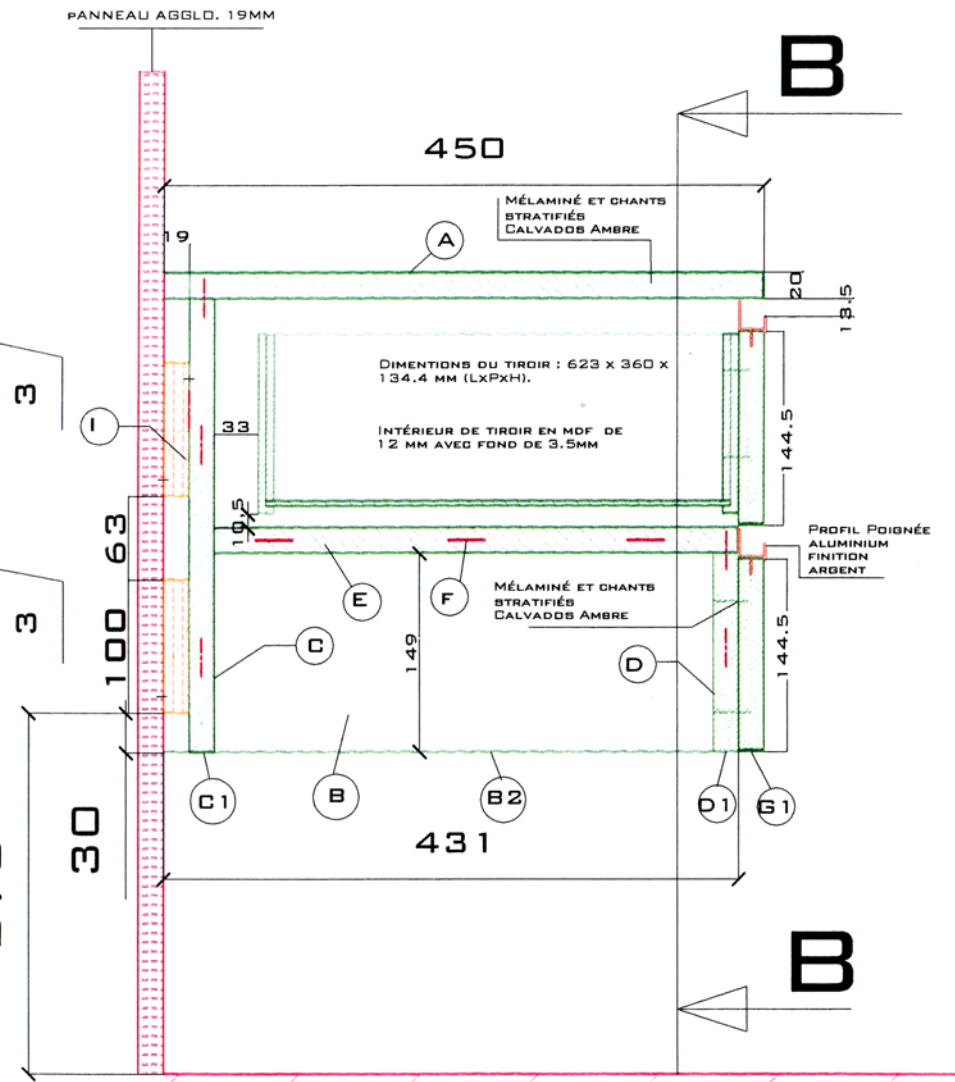
COUPE A-A
