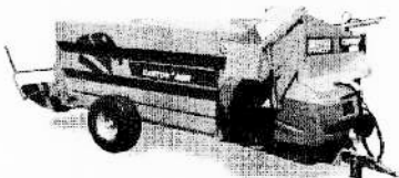
CASTOR+ 60 RC Capacité de chargement : En transport : 3 balles rondes Ø 1,80 m ou 2 bigs longueur 2,50 m. En distribution : 2 balles rondes Ø 1,80 m ou 2 bigs longueur 2,50 m.
