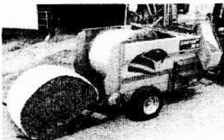
CASTOR+ 30 RC Machine équipée en série d'une porte arrière ramasseuse, pilotée depuis la cabine du tracteur ou depuis un deuxième poste de commande, à l'arrière de la machine (option). Commande "confort" avec sécurité du tapis de fond intégrée. Circuits hydrauliques protégés par un filtre pression, à l'entrée de la machine, pour prévenir tout risque de pollution par les huiles du tracteur.
