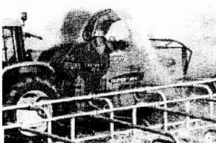
CASTOR+ 30 RUT Machine équipée en série d'une goulotte universelle (U) et d'une porte arrière ramasseuse (R), pilotée depuis la cabine du tracteur par des commandes "téléflexibles".
