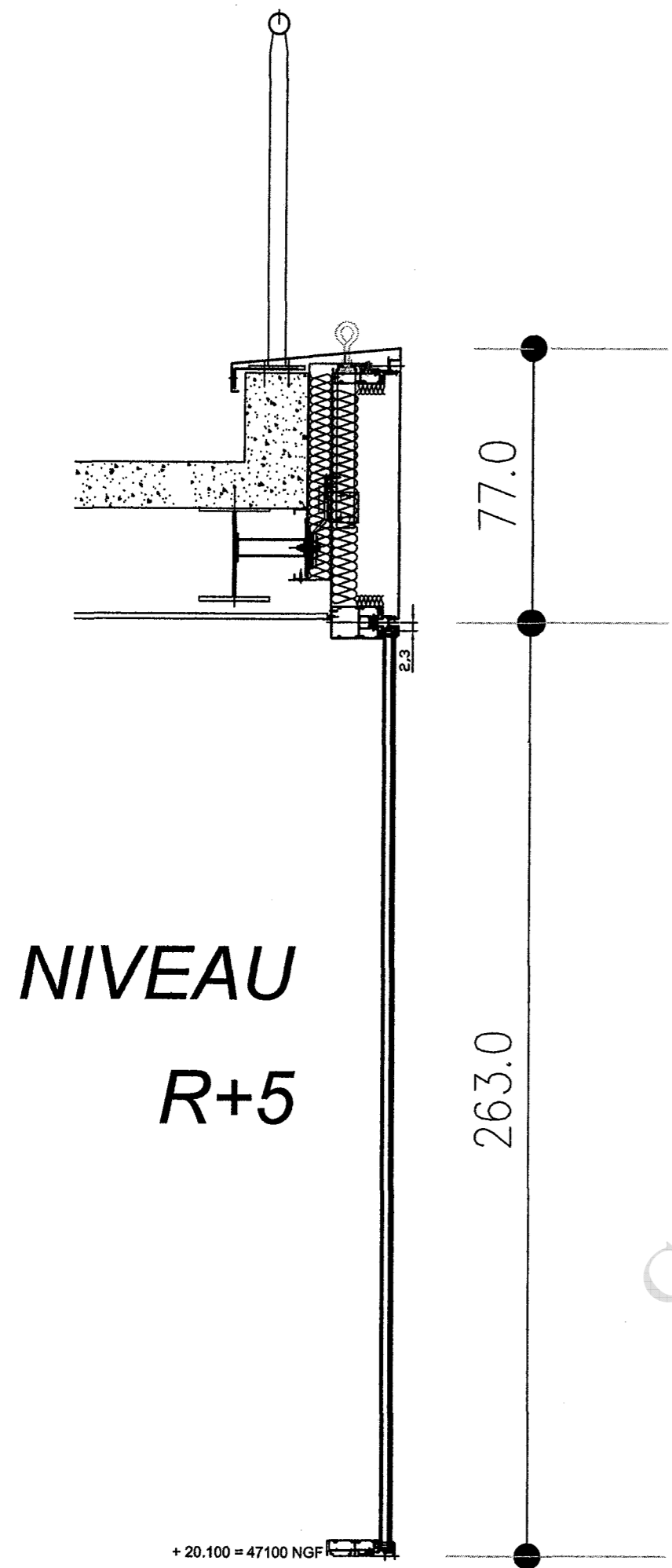
COUPE VERTICALE (COTES EN CM)
