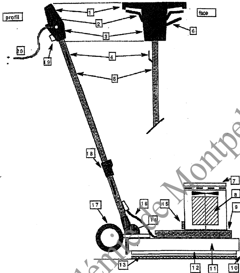
Schéma descriptif de la monobrosse
