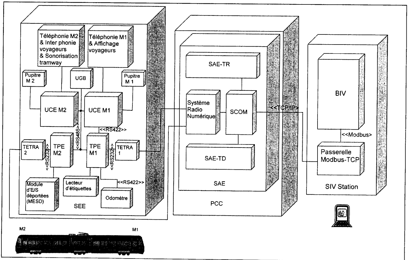
Diagramme des nœuds du SAEIV
