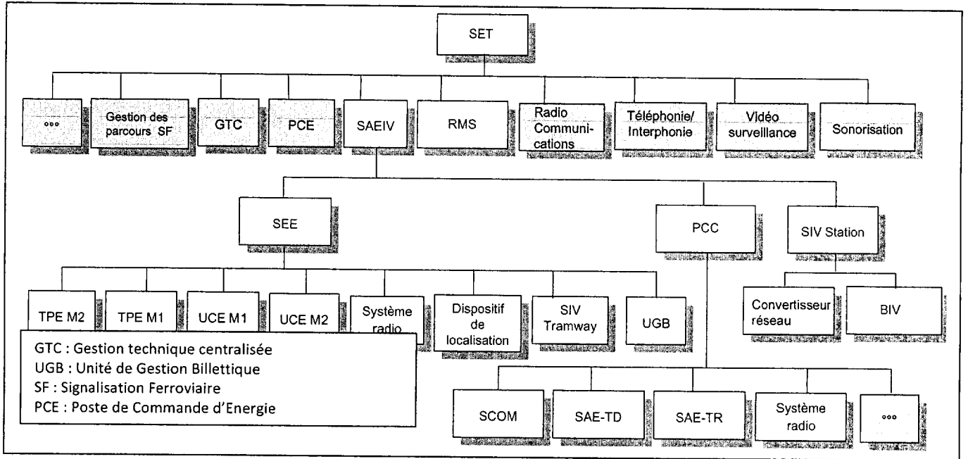
Principaux sous-systèmes et fonctions du Système d'Exploitation du Tramway (SET)
