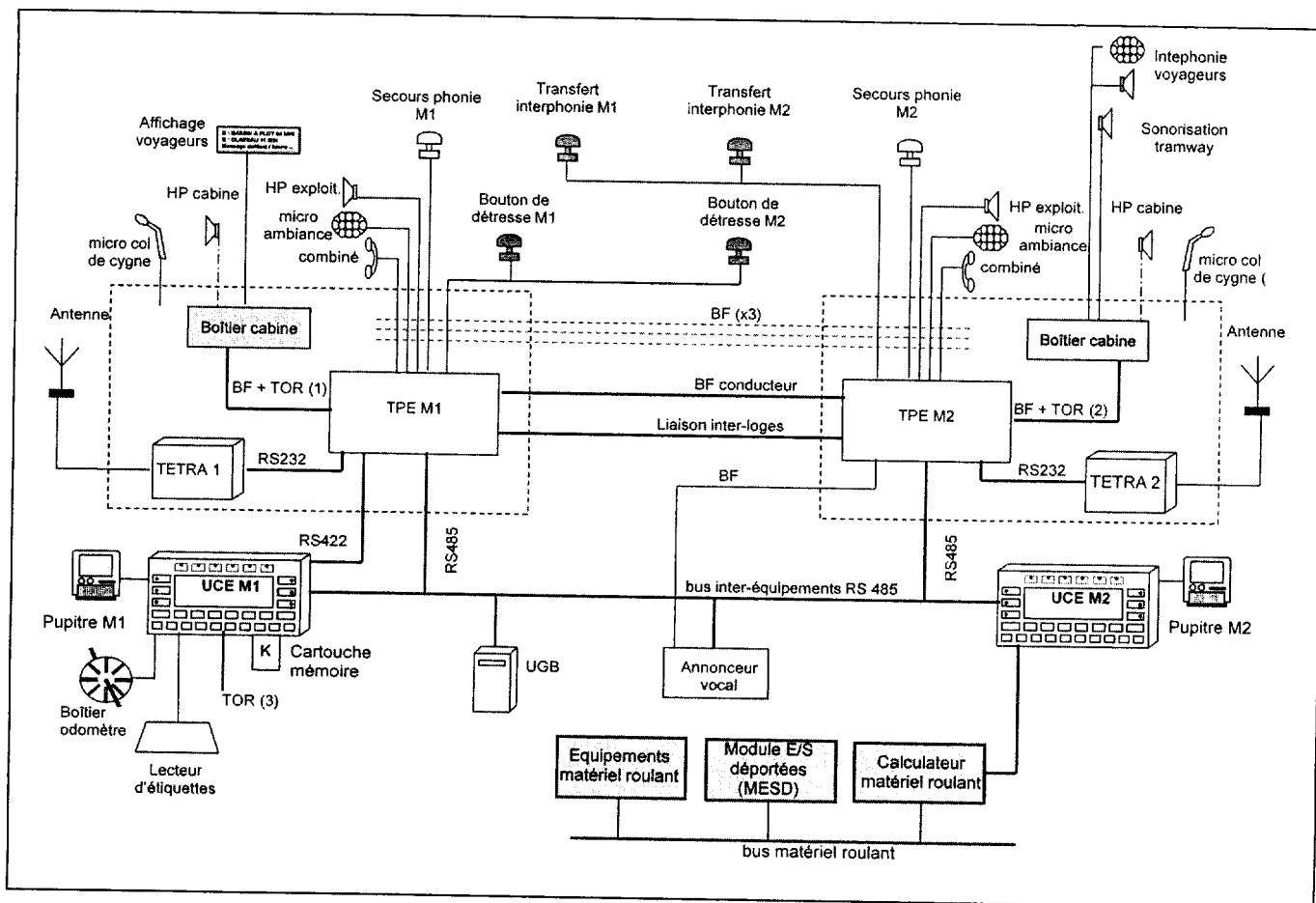
Architecture générale du Système d'Exploitation Embarqué (SEE)
