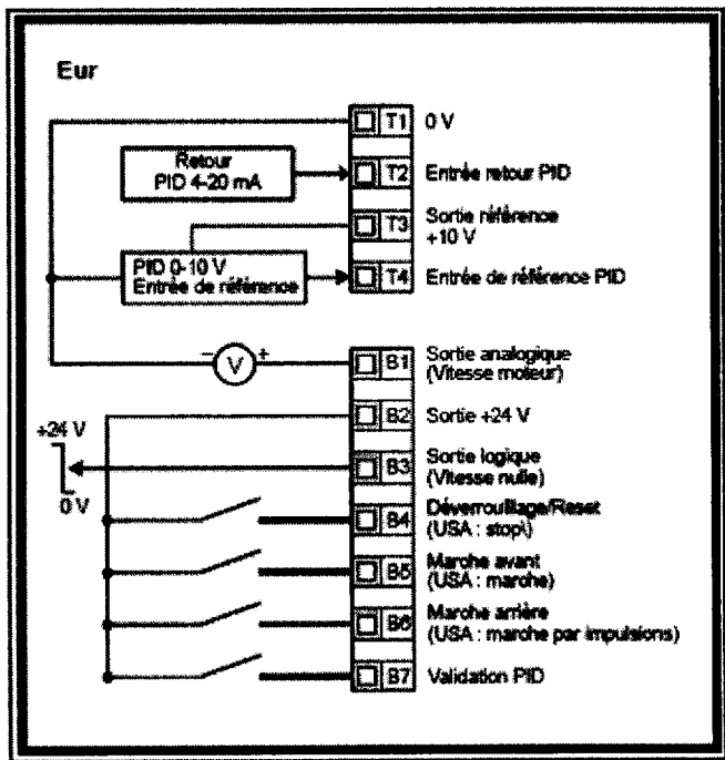
Raccordement de commande du variateur
