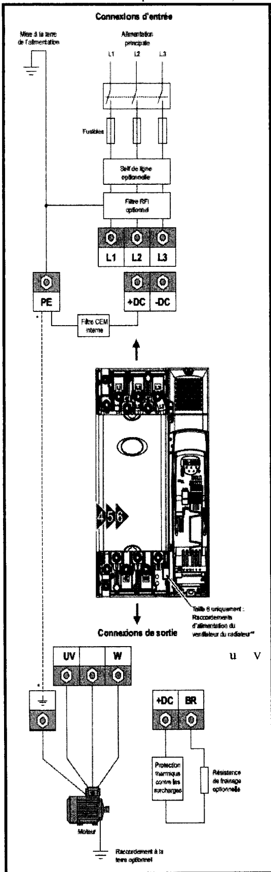
Illustration 4-3 Raccordement de puissance des tailles 4, 5 et 6
