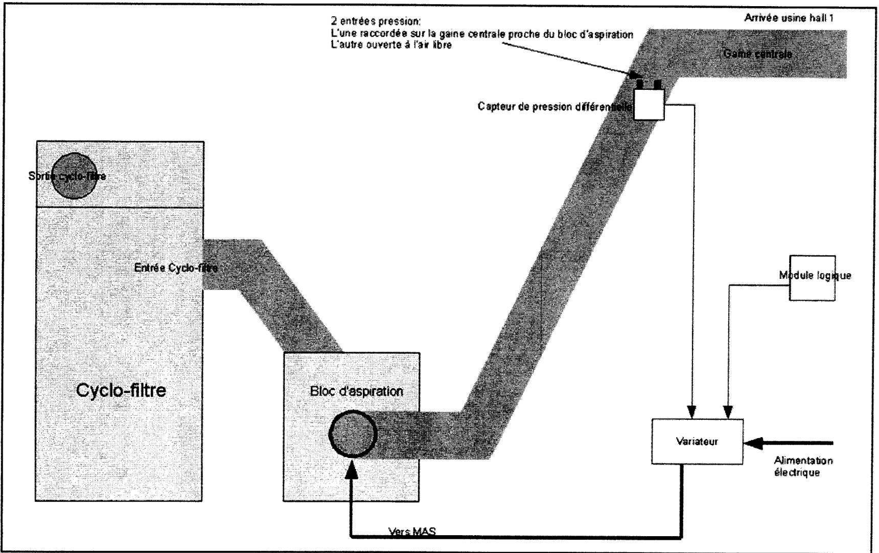
Synoptique du système d'aspiration
