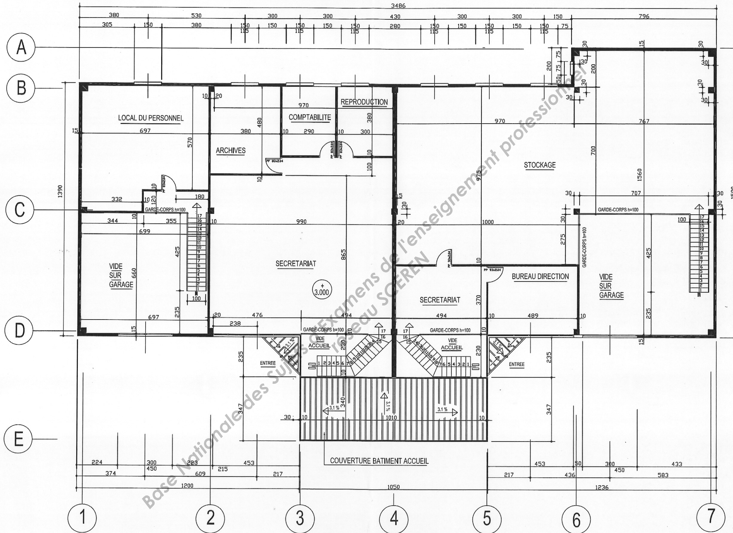
PLAN ETAGE
