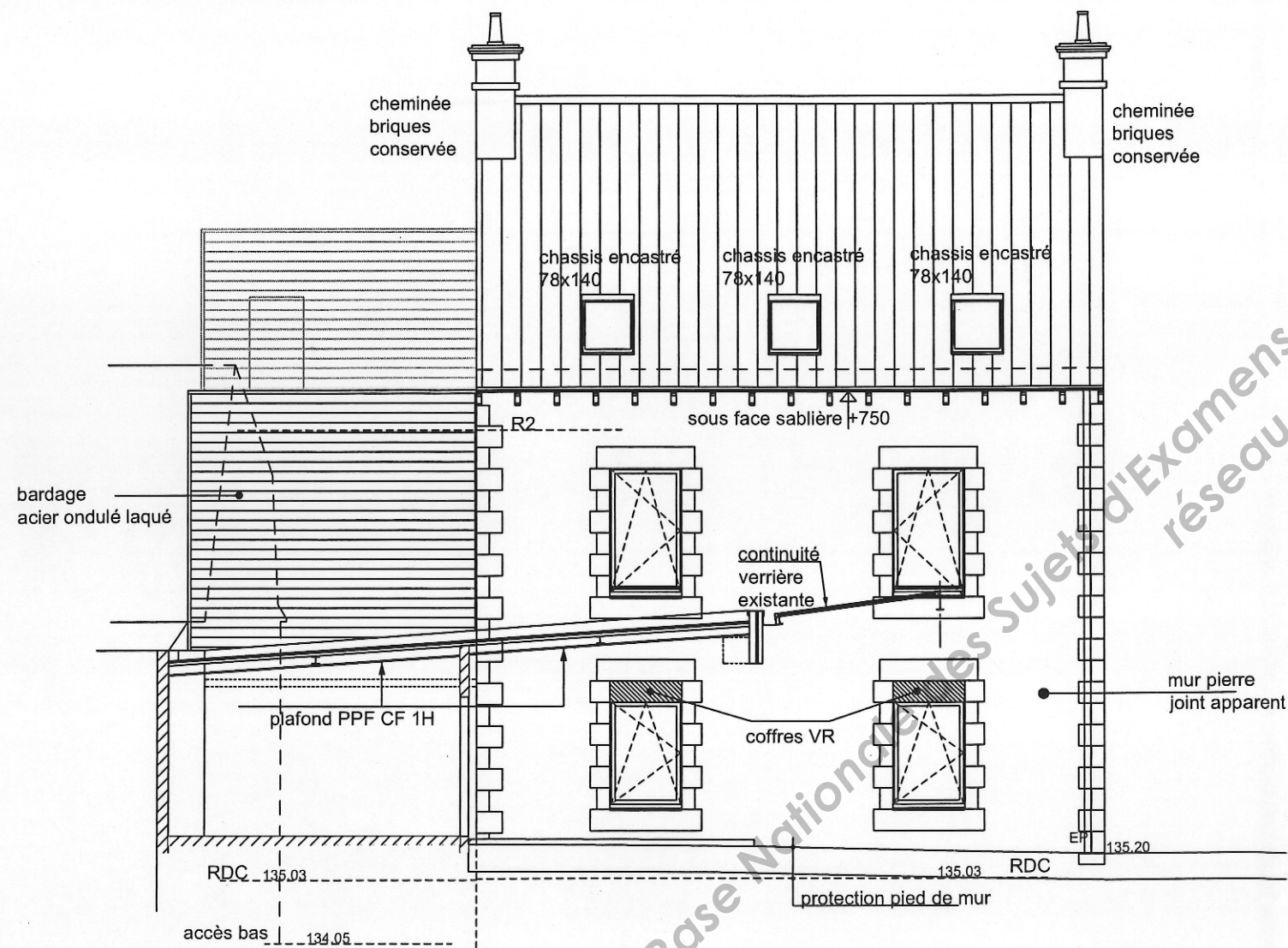
ELEVATION NORD
