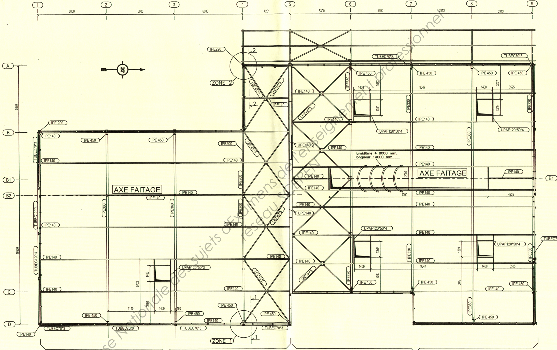
HALL 1: ESPACE DE VENTE niveau faitage : + 6450 pente 3%
