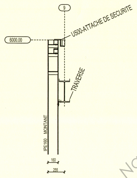
COUPE DE PRINCIPE SUR ACROTERE FILE 9
