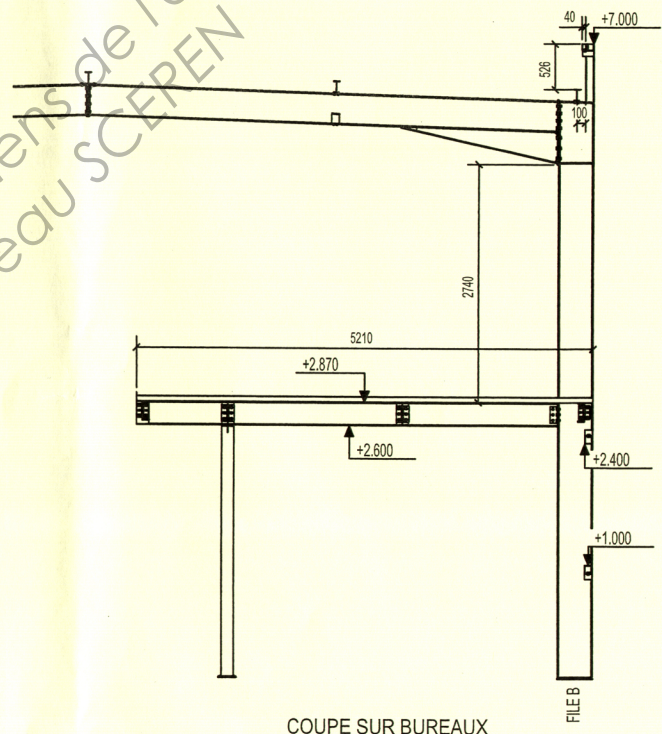
COUPE SUR BUREAUX
