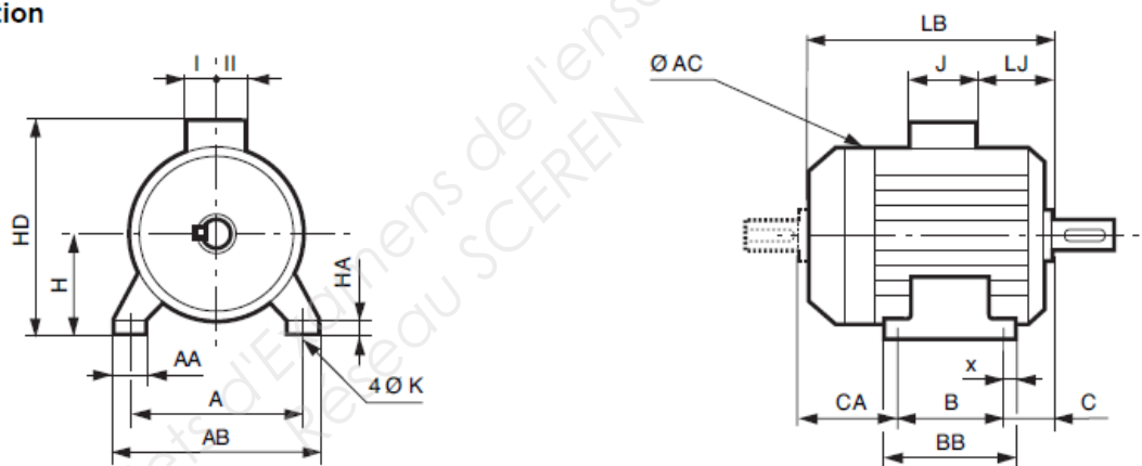
Dimensions principales (en mm)
