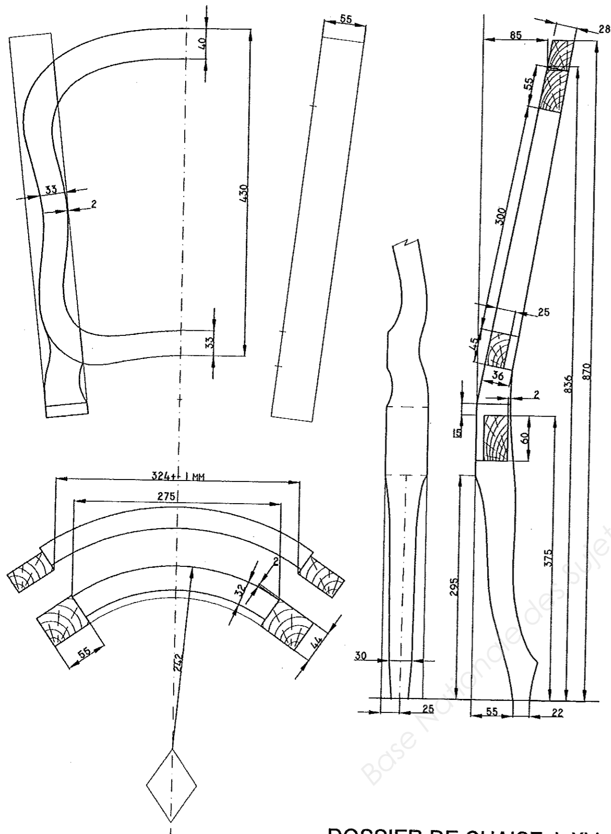
DOSSIER DE CHAISE L XV "en cabriolet" Ech : 1/5
