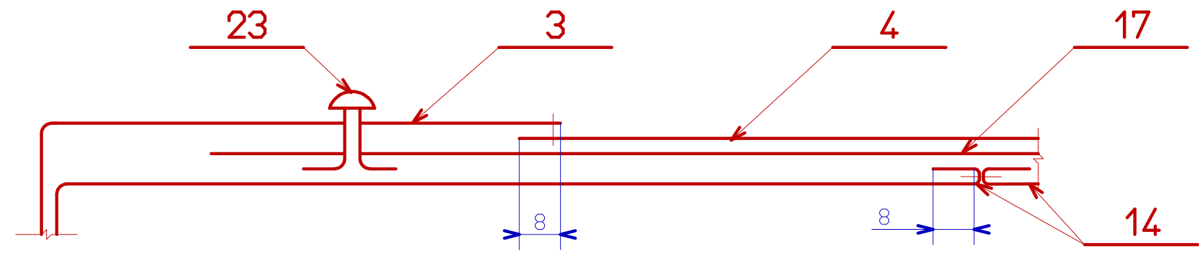
A-A vue de dessous
