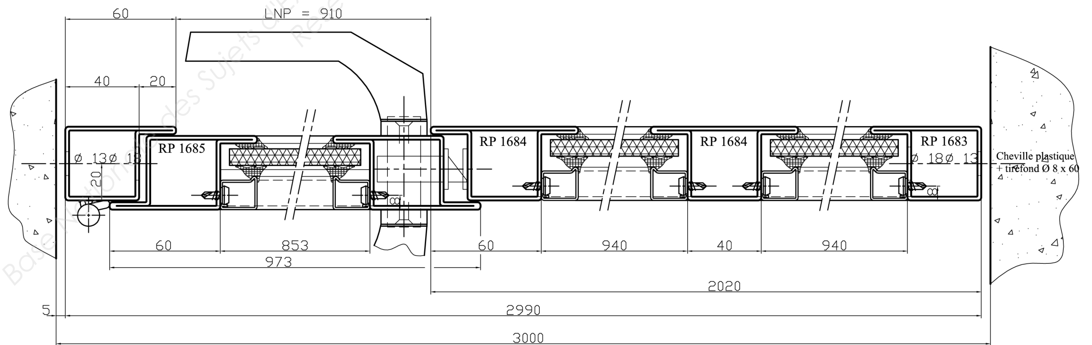
COUPE A-A
